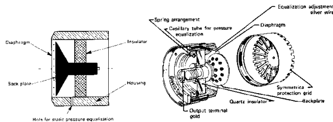
شکل شماره ۵- نمایی از ساختار میکروفن خازنی
