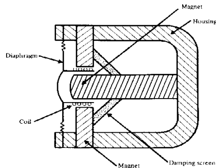
شکل شماره ۴- نمایشی از ساختار میکروفن دینامیک
