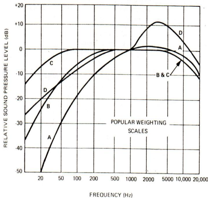
نمودار شماره ۱-منحنی تصحیح در هر شبکه توزین فرکانس
