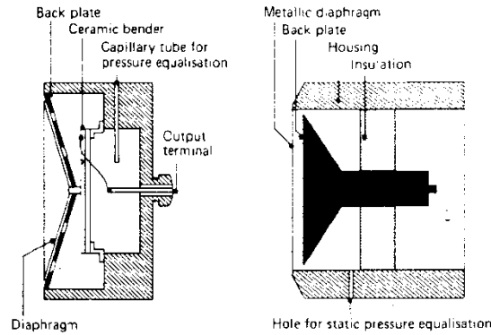
شکل شماره ۲- نمایشی از ساختار میکروفن کریستالی
