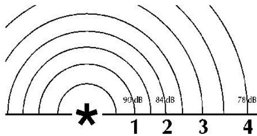
شکل شماره ۸ - تاثیر فاصله در کاهش تراز فشار صوت در میدانهای آزاد
