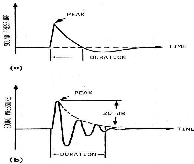
شکل شماره ۷- انواع صدا های لحظه ای (a: صدای ضربه ای- b: صدای کوبه ای)
