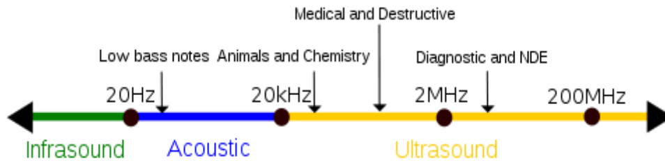
شکل شماره ۲ - نمایشی از طیف فرکانسی صوت
