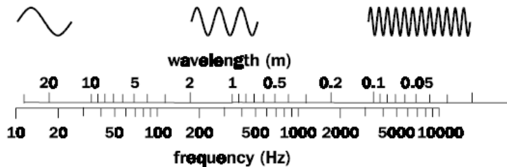
شکل شماره ۱- نمایش اشکال طول موج در فرکانسهای مختلف
