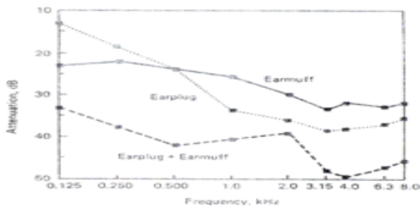
نمودار شماره ۲- تأثیر استفاده مجزا از حفاظ گوش نوع ایرپلاگ، ایرماف و استفاده توأم آنها در افت انتقال
