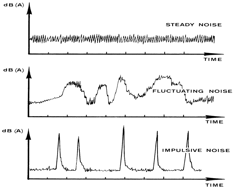
شکل شماره ۶- انواع صدا های پیوسته
