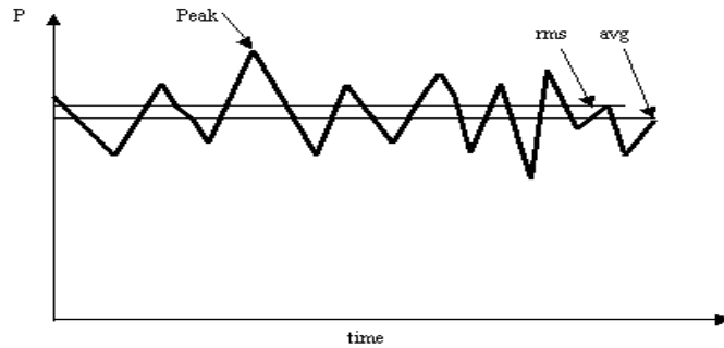
شکل شماره ۵- مقایر حداکثر، مؤثر و میانگین فشارها در يك دوره زمانی
